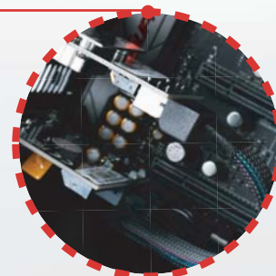
Mini-SAS 어댑터와 전원 어댑터의 내부 케이블을 연결합니다
